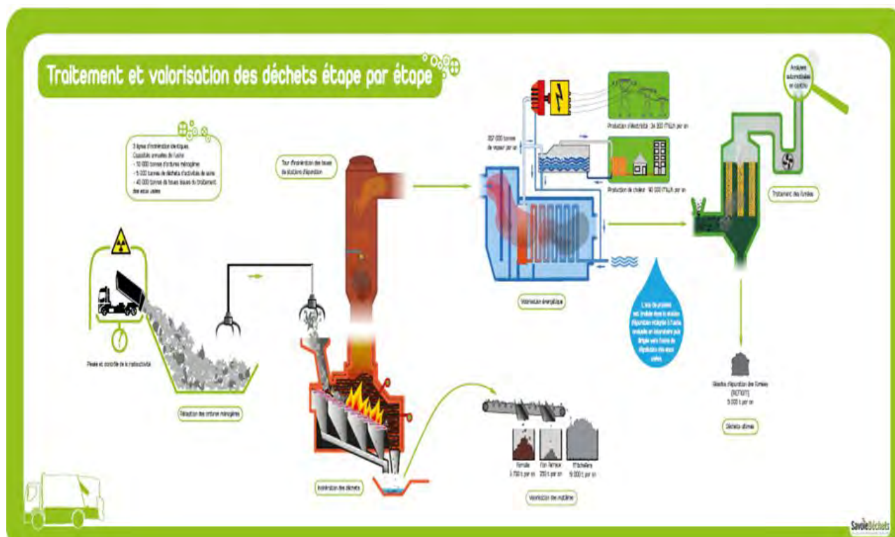
Schéma 1 : Fonctionnement de l'UVETD de Chambéry
